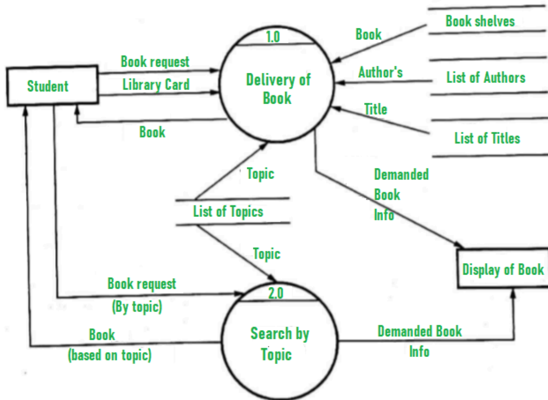
Level 1 DFD
